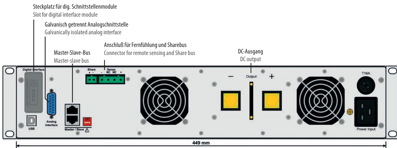
Rückansicht Standardmodell
